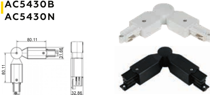
Cylinder Conector Flex Blanco / Negro / Plástico Inyectado Voltaje: 480 V~ IP 40 - IK 6 - 1 Kg
